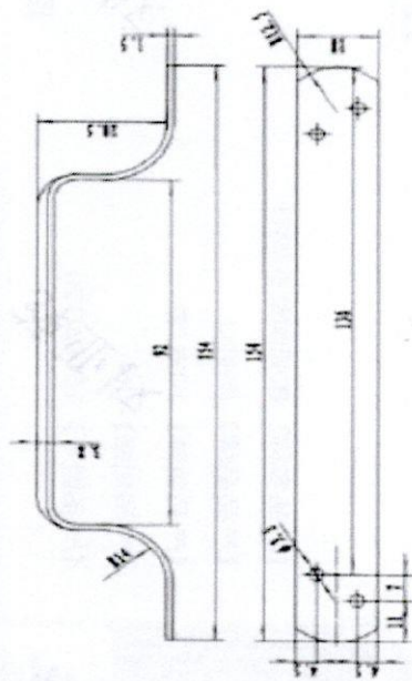
图 1 把手规格及样式图
